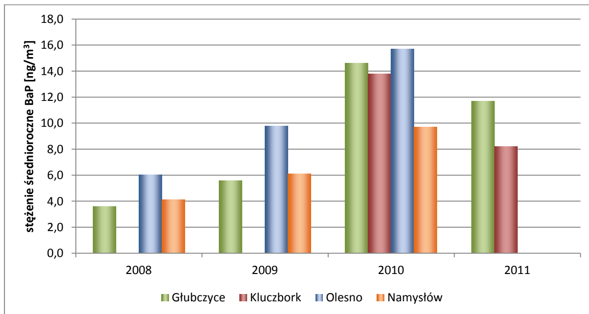
Rysunek 13. Wartości stężeń średniorocznych benzo(a)pirenu zarejestrowanych na stacjach pomiarowych zlokalizowanych w strefie opolskiej w latach 2008-2011 51
