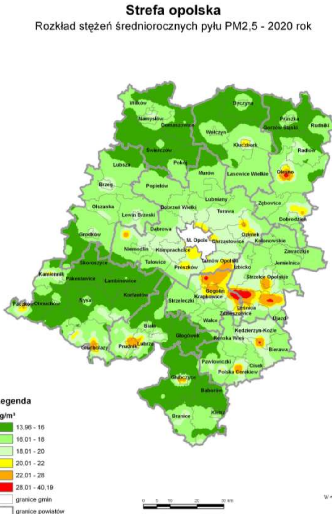
Rysunek 25. Rozkład stężeń średniorocznych pyłu PM 2,5 na obszarze strefy opolskiej w roku prognozy 2020 76
