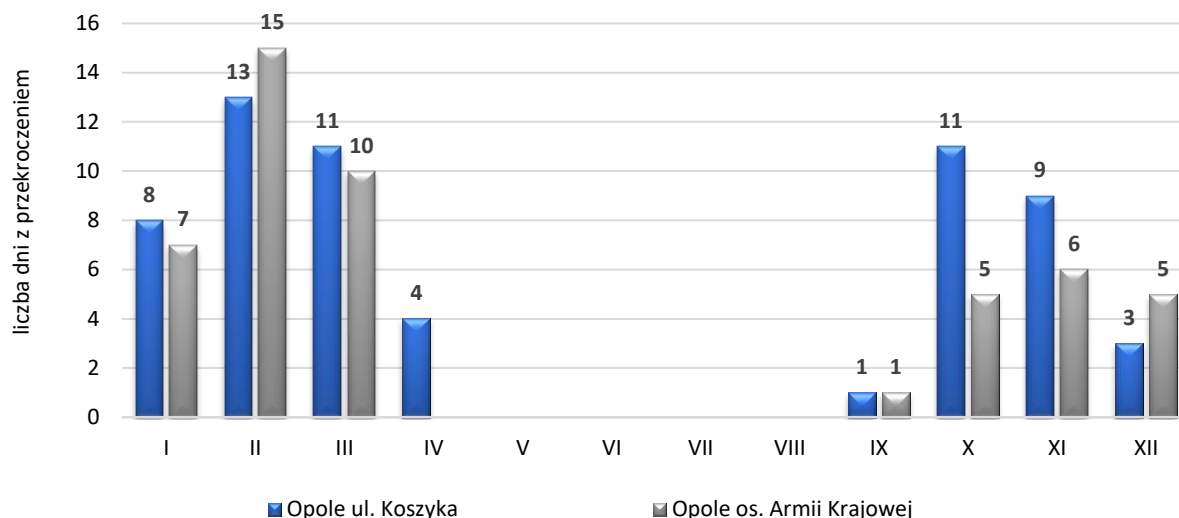
Rysunek 12. Liczba dni w poszczególnych miesiącach z przekroczeniem poziomu dopuszczalnego 24-godzinny pyłu zawieszony PM10 w roku 2018 w punktach pomiarowych w strefie miasto Opole 66
