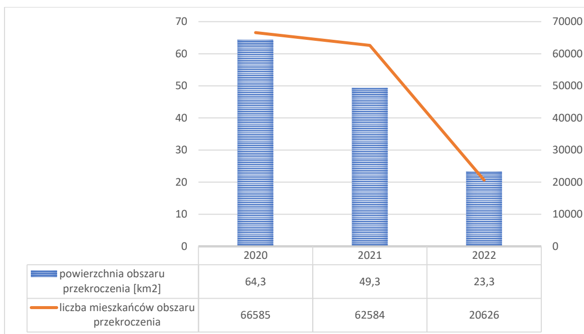
Rysunek 1 Powiercznia obszaru przekroczeń i liczba mieszkańców obszaru przekroczenia, objęta zanieczyszczeniem dla kryterium: Pył zawieszony PM 10 . Typ normy – poziom dopuszczalny. Czas uśrednienia: średnia 24 godz.
