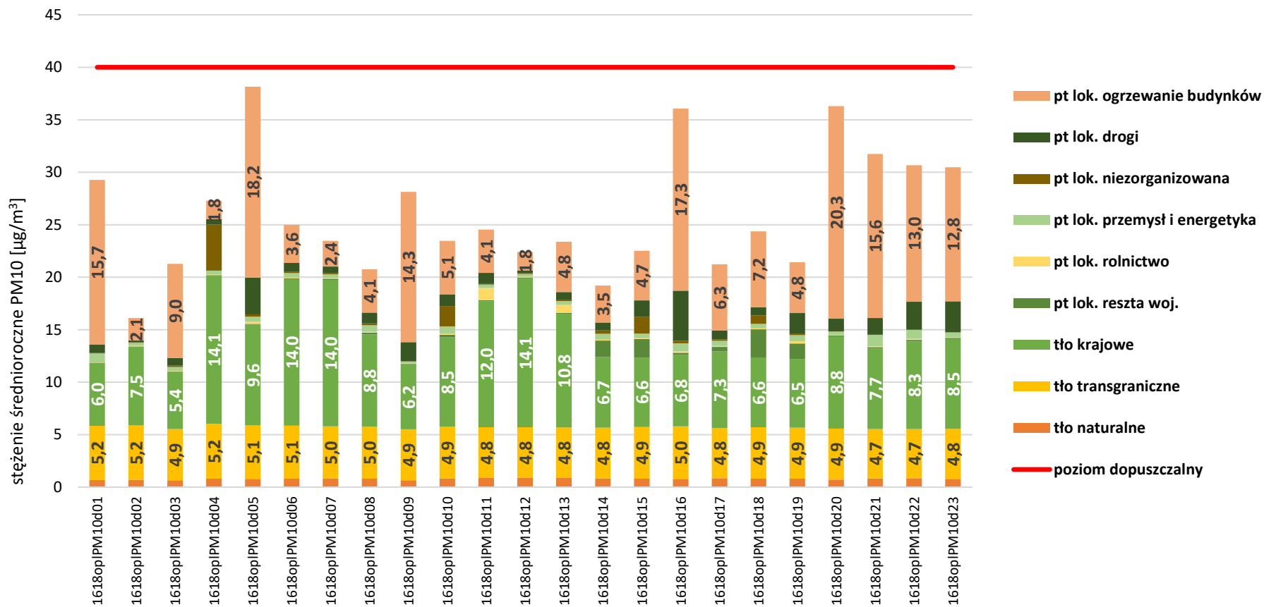
Rysunek 32. Prezentacja poziomów tła regionalnego oraz lokalnego przyrostu stężeń dla pyłu zawieszonego PM10 w obszarach przekroczeń w strefie opolskiej w 2018 roku 113
