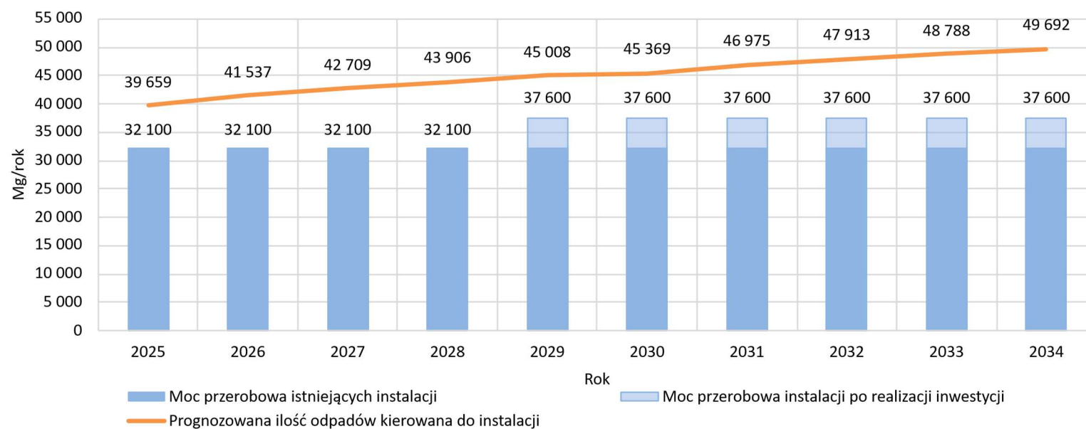
Rysunek 43. Bilans przepustowości instalacji do recyklingu szkła na terenie województwa opolskiego
