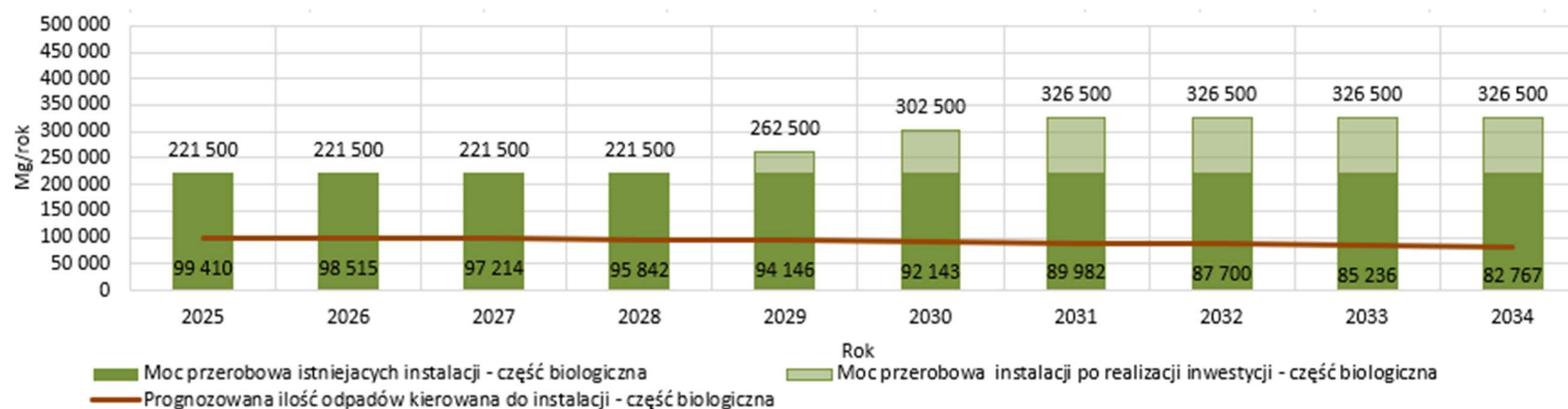
Rysunek 47. Bilans przepustowości instalacji MBP na terenie województwa opolskiego przed i po realizacji inwestycji – część biologiczna
