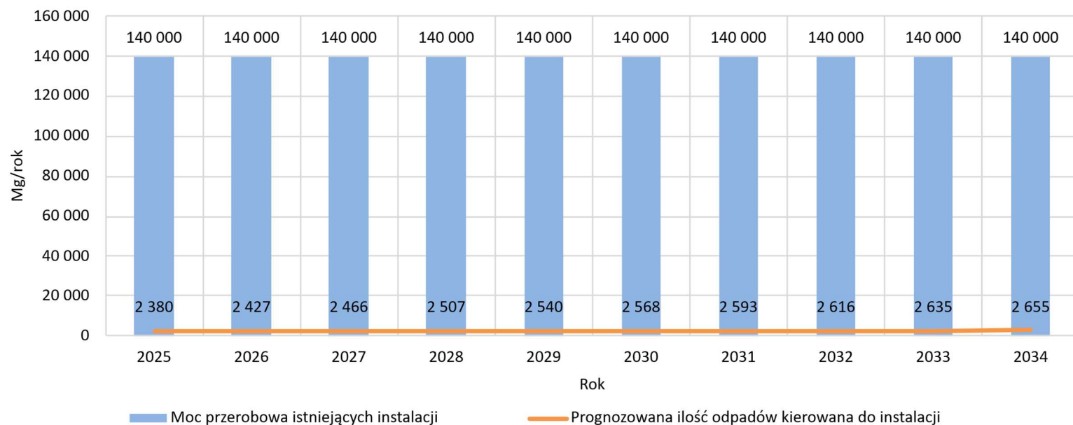
Rysunek 39. Bilans przepustowości instalacji do recyklingu drewna na terenie województwa opolskiego
