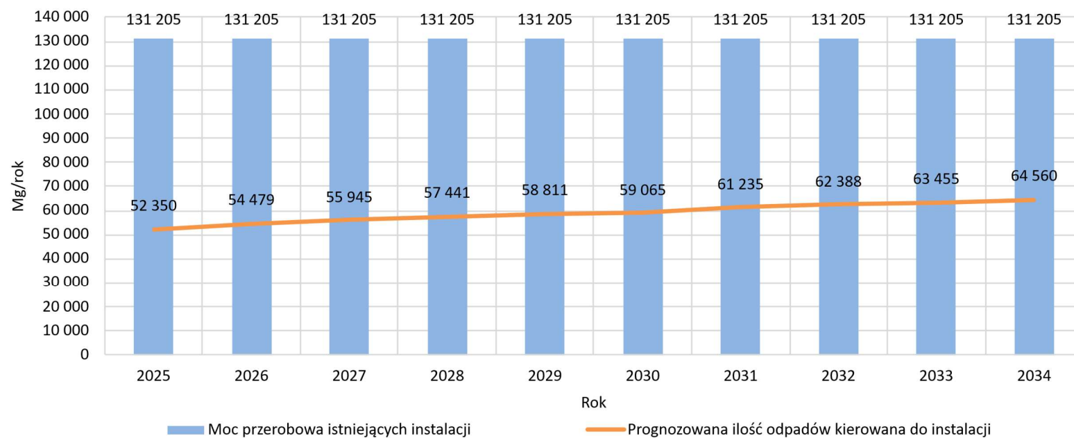
Rysunek 42. Bilans przepustowości instalacji do recyklingu papieru na terenie województwa opolskiego
