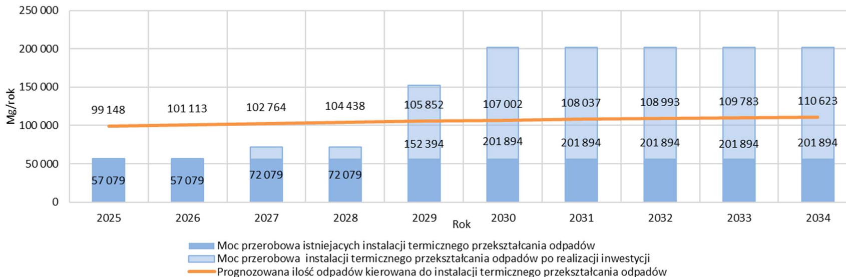
Rysunek 49. Bilans przepustowości instalacji do termicznego przekształcania odpadów komunalnych na terenie województwa opolskiego
