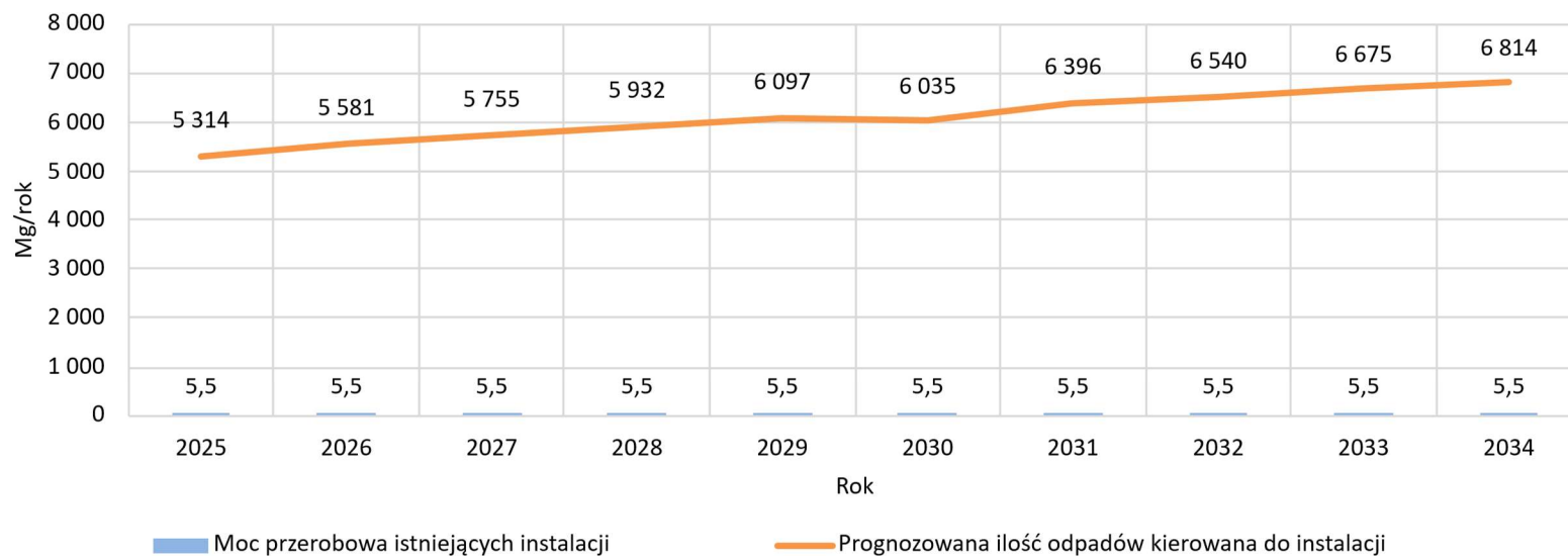
Rysunek 40. Bilans przepustowości instalacji do recyklingu metali żelaznych na terenie województwa opolskiego
