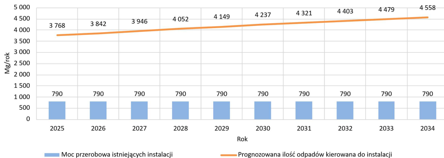
Rysunek 41. Bilans przepustowości instalacji do recyklingu metali nieżelaznych na terenie województwa opolskiego
