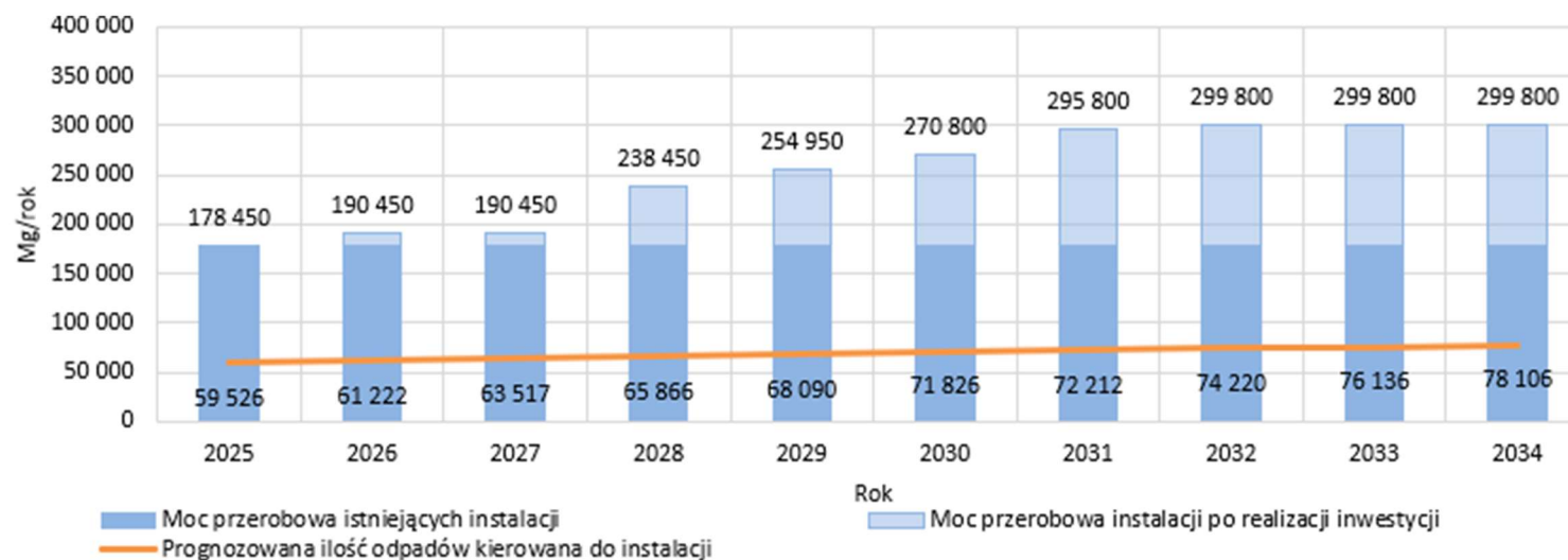
Rysunek 37. Bilans przepustowości instalacji do bioodpadów przed i po realizacji inwestycji na terenie województwa opolskiego
