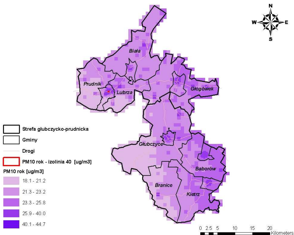
Rysunek 78. Rozkład stężeń pyłu zawieszonego PM 10 o okresie uśredniania wyników pomiarów rok kalendarzowy z emisji całkowitej na terenie strefy głubczycko-prudnickiej w 2008r.
