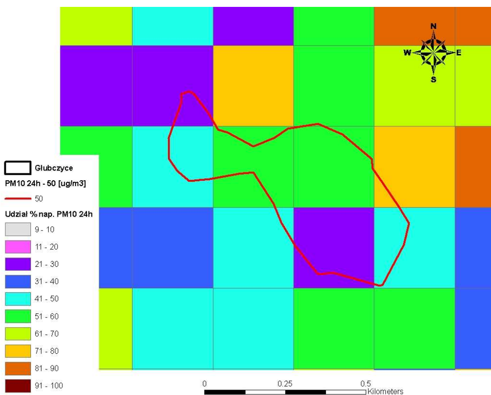
Rysunek 90. Udział procentowy emisji napływowej w imisji całkowitej pyłu zawieszonego PM 10 o okresie uśredniania wyników pomiarów 24 godziny (36 max) w Głubczycach
