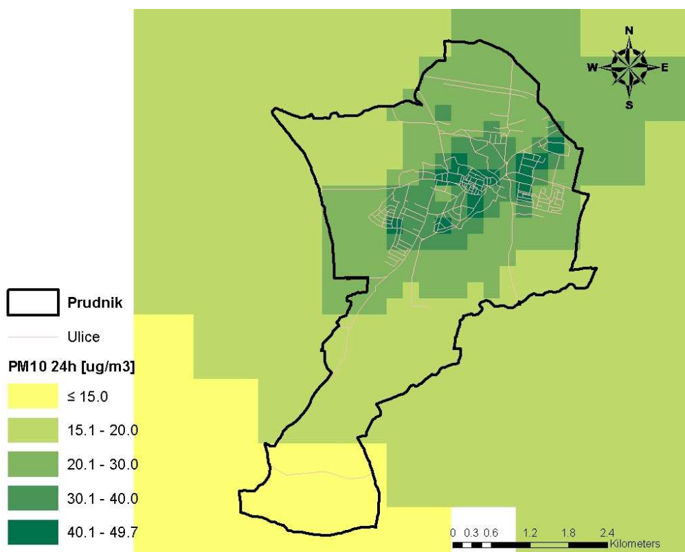
Rysunek 117. Rozkład stężeń pyłu zawieszonego PM 10 o okresie uśredniania wyników pomiarów 24 godziny pochodzących od całkowitej emisji, po zastosowaniu działań naprawczych oraz odjęciu napływu transgranicznego i stężeń pochodzących od emisji naturalnej
