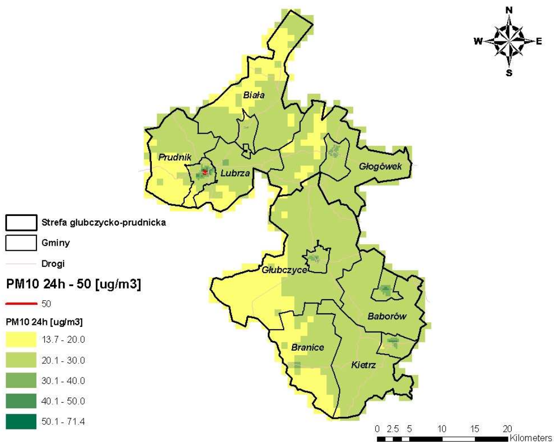
Rysunek 112. Rozkład stężeń pyłu zawieszonego PM 10 o okresie uśredniania wyników pomiarów 24 godziny (36 max) z emisji całkowitej na terenie strefy głubczycko-prudnickiej w 2008 r. po odjęciu napływu transgranicznego i stężeń pochodzących od emisji naturalnej
