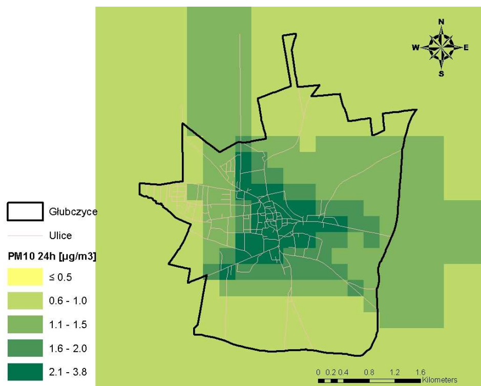
Rysunek 118. Rozkład stężeń pyłu zawieszonego PM 10 o okresie uśredniania wyników pomiarów 24 godziny pochodzących od emisji liniowej, po zastosowaniu działań naprawczych w Głubczycach
