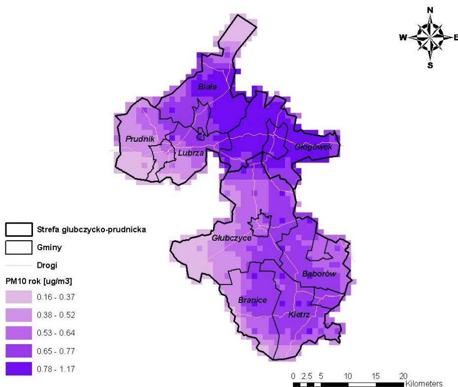
Rysunek 68. Rozkład stężeń pyłu zawieszonego PM 10 o okresie uśredniania wyników pomiarów rok kalendarzowy pochodzących z rolnictwa na terenie strefy głubczycko-prudnickiej w 2008 r.
