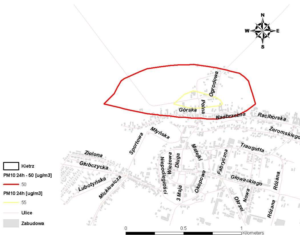
Rysunek 95. Obszar przekroczeń poziomu dopuszczalnych stężeń pyłu zawieszonego PM 10 o okresie uśredniania wyników pomiarów 24 godziny (36 max) w Kietrz
