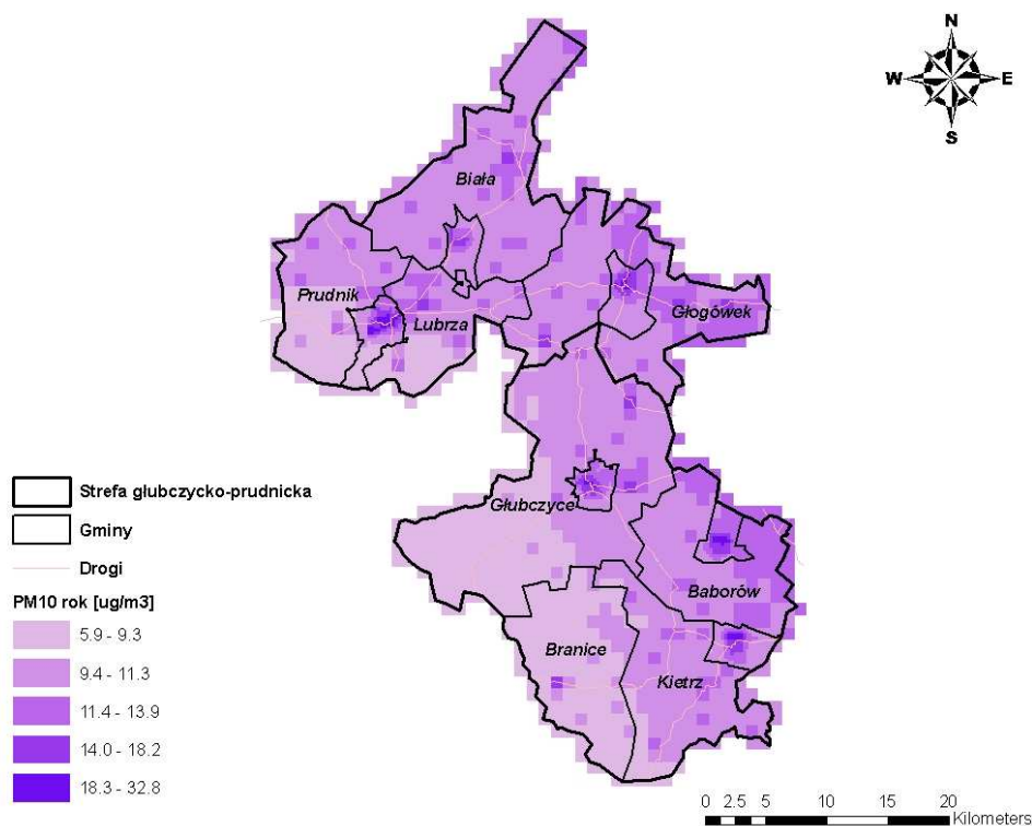
Rysunek 114. Rozkład stężeń pyłu zawieszonego PM 10 o okresie uśredniania wyników pomiarów rok kalendarzowy z emisji całkowitej na terenie strefy głubczycko-prudnickiej w 2008 r. po odjęciu napływu transgranicznego i stężeń pochodzących od emisji naturalnej
