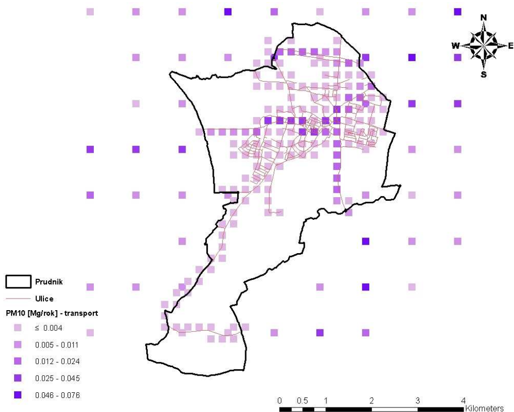
Rysunek 42. Emisja pyłu zawieszonego PM 10 z tarcia, ze źródeł komunikacyjnych w Prudniku w 2008 r.
