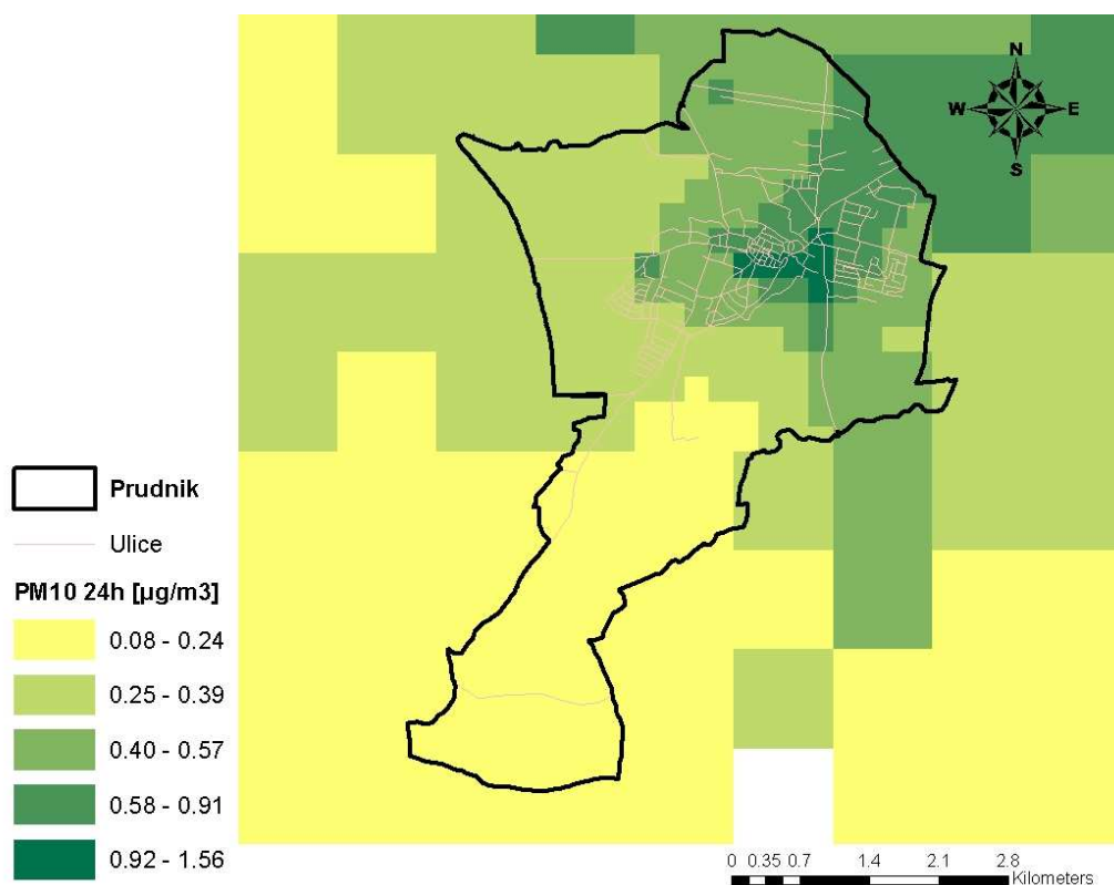
Rysunek 116. Rozkład stężeń pyłu zawieszonego PM 10 o okresie uśredniania wyników pomiarów 24 godziny pochodzących od emisji liniowej , po zastosowaniu działań w zakresie komunikacji w Prudniku
