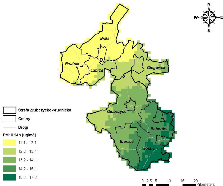
Rysunek 47. Stężenia pyłu zawieszonego PM 10 o okresie uśredniania wyników pomiarów 24 godziny (36 max) w strefie głubczycko-prudnickiej pochodzące od napływu transgranicznego w 2008 r.
