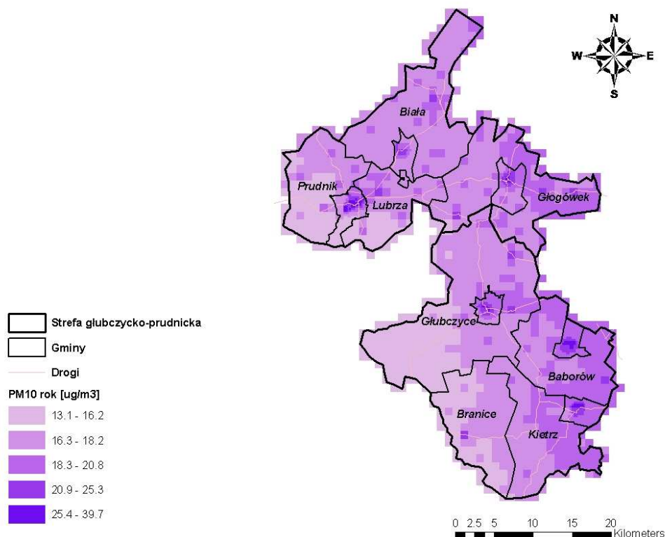
Rysunek 111. Rozkład stężeń pyłu zawieszonego PM 10 o okresie uśredniania wyników pomiarów rok kalendarzowy z emisji całkowitej na terenie strefy głubczycko-prudnickiej w 2008 r. po odjęciu stężeń pochodzących od emisji naturalnej
