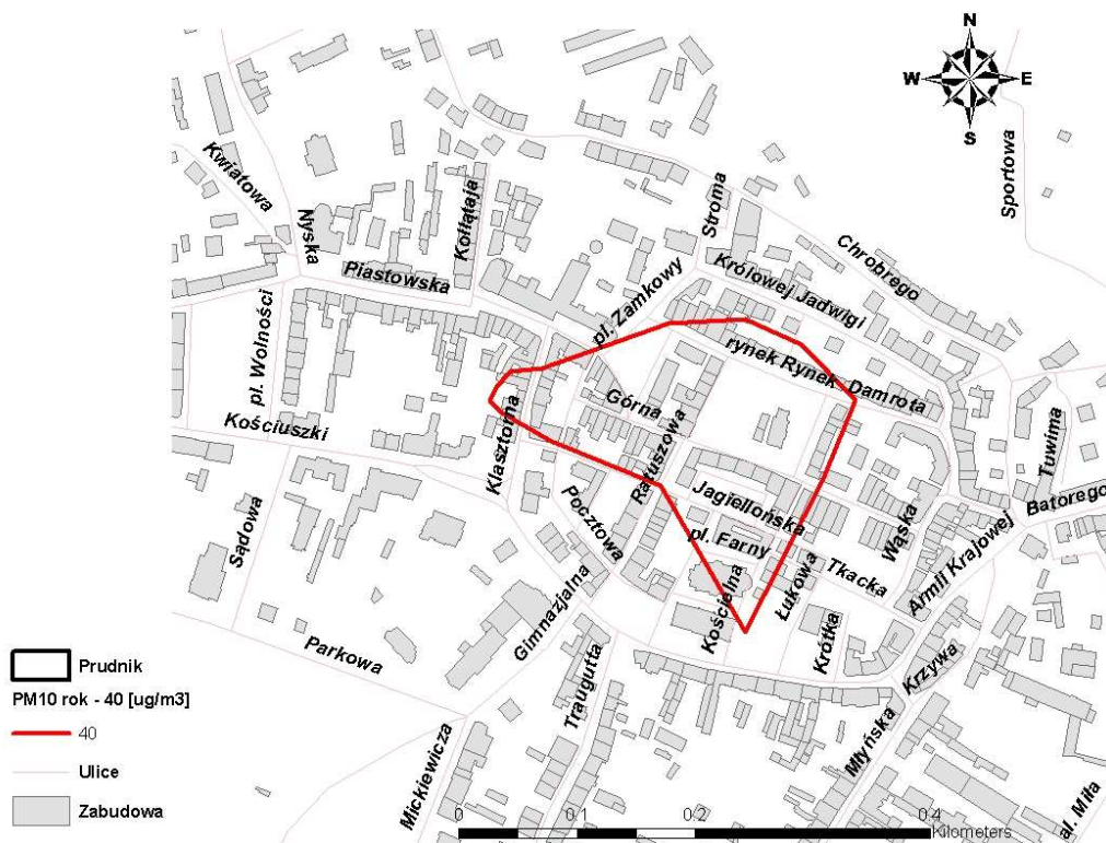
Rysunek 105. Obszar przekroczeń poziomu dopuszczalnego stężenia pyłu zawieszonego PM 10 o okresie uśredniania wyników pomiarów rok kalendarzowy w Prudniku
