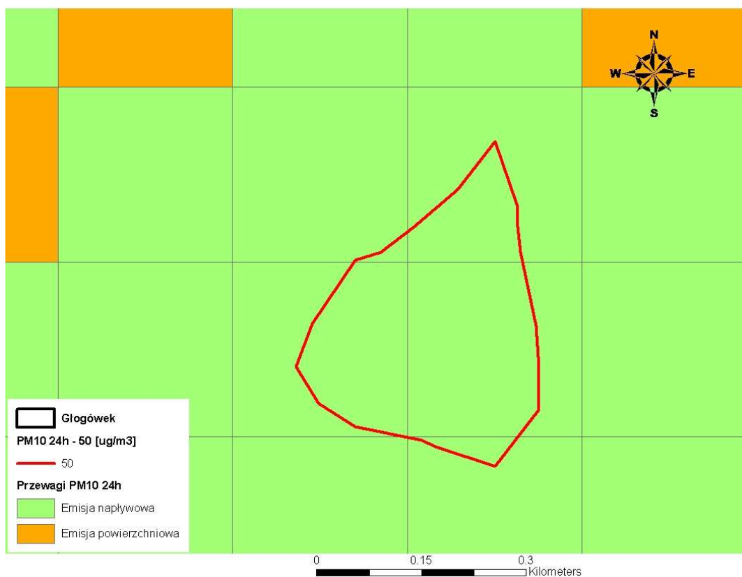
Rysunek 92. Większościowy udział poszczególnych typów emisji w imisji pyłu zawieszonoego PM 10 o okresie uśredniania wyników pomiarów 24 godziny (36 max) w Głogówku
