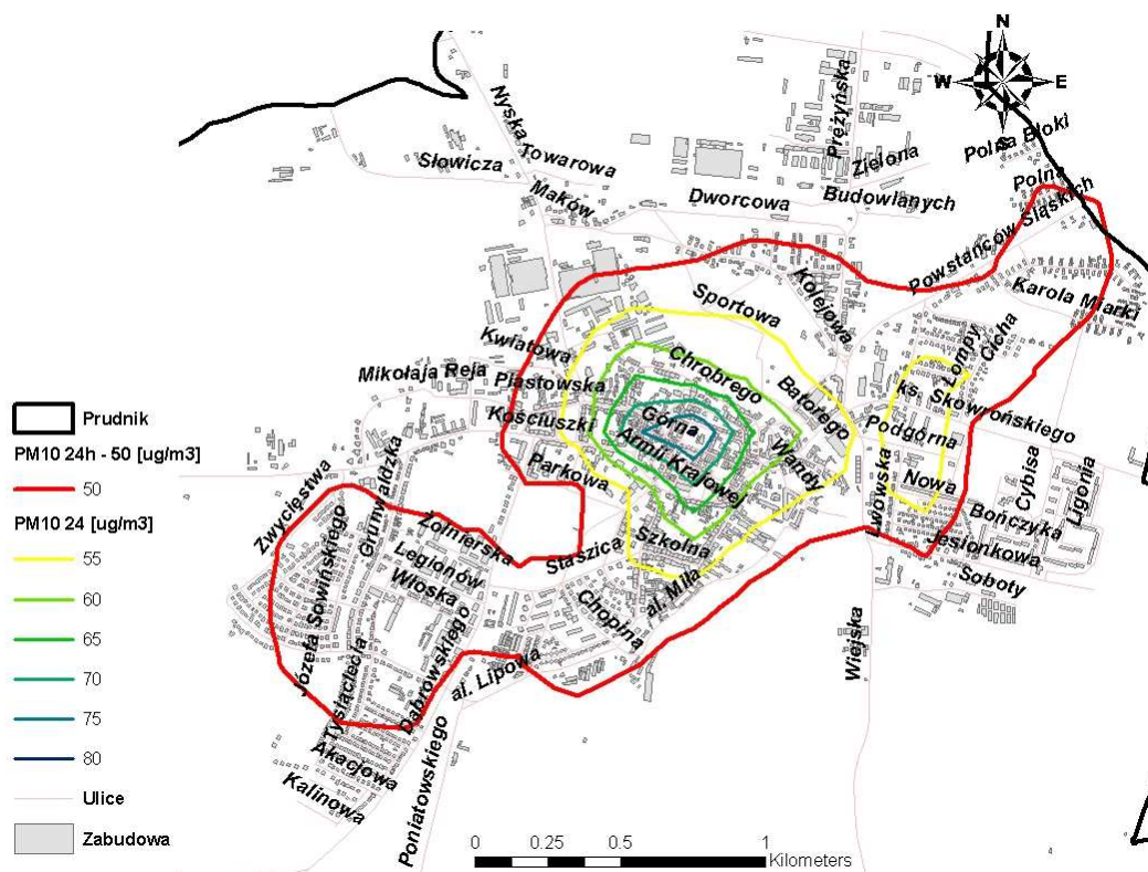
Rysunek 82. Obszar przekroczeń poziomu dopuszczalnych stężeń pyłu zawieszonego PM 10 o okresie uśredniania wyników pomiarów 24 godziny (36 max) w Prudniku
