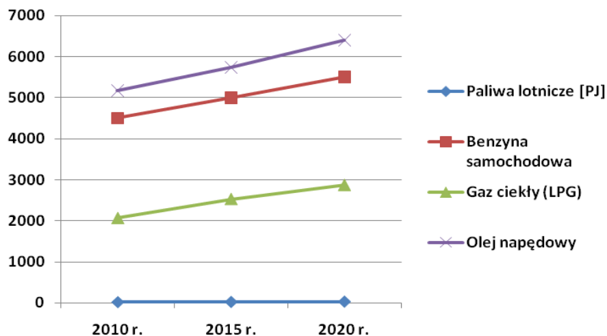
Rysunek 121. Prognoza spalania paliw [Gg] w transporcie do roku 2020
