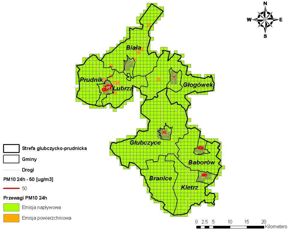
Rysunek 75. Udziały poszczególnych typów emisji w stężeniach pyłu zawieszonego PM 10 o okresie uśredniania wyników pomiarów 24 godziny (36 max) na terenie strefy głubczycko-prudnickiej w 2008 r.
