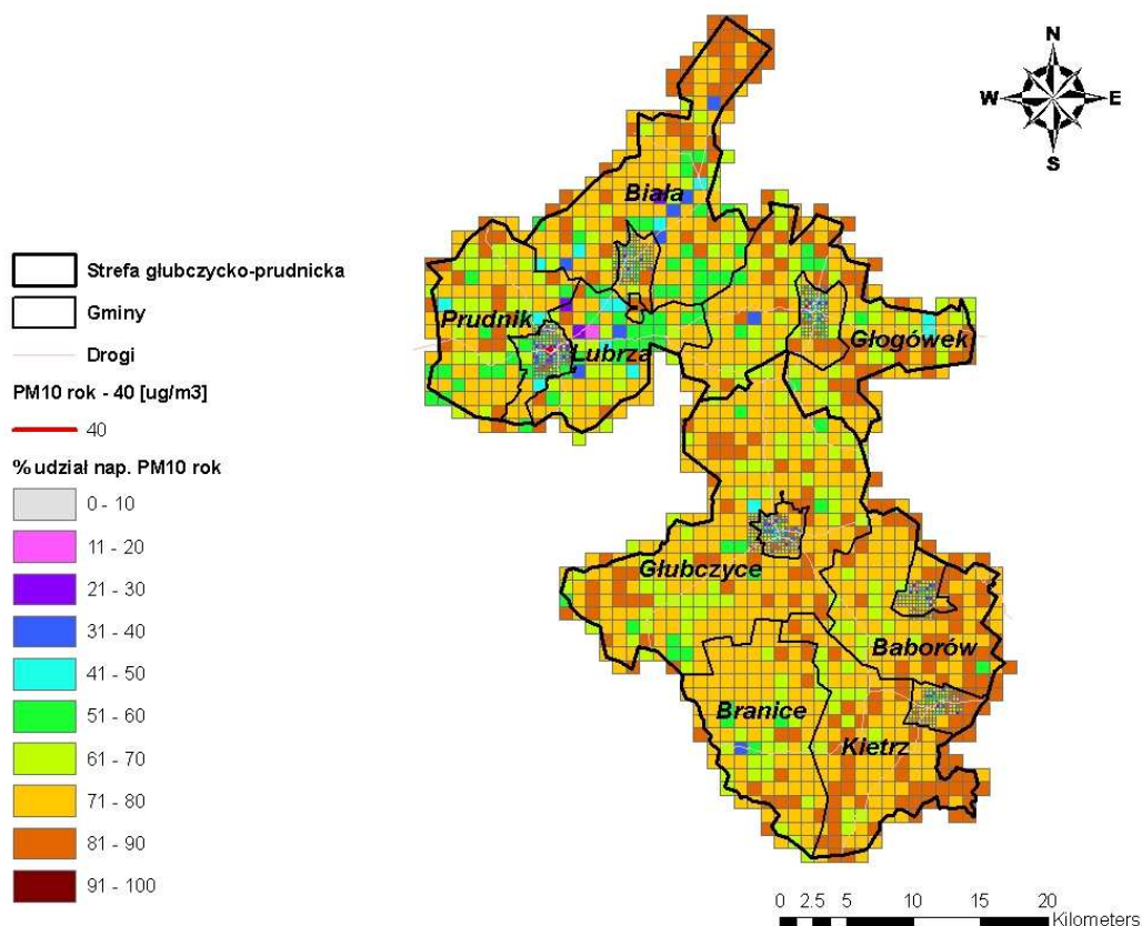
Rysunek 81. Procentowy udział emisji napływowej w stężeniach pyłu zawieszzonego PM 10 o okresie uśredniania wyników pomiarów rok kalendarzowy na terenie strefy głubczycko-prudnickiej w 2008 r.
