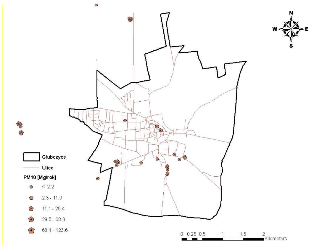
Rysunek 29. Emisja pyłu zawieszonego PM 10 z emitorów punktowych na terenie Głubczyca w 2008 r.
