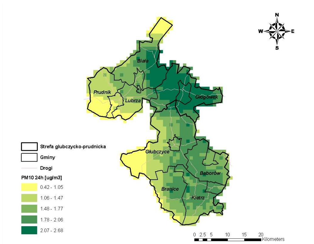
Rysunek 67. Rozkład stężeń pyłu zawieszonego PM 10 o okresie uśredniania wyników pomiarów 24 godziny (36 max) pochodzących z rolnictwa na terenie strefy głubczycko-prudnickiej w 2008 r.
