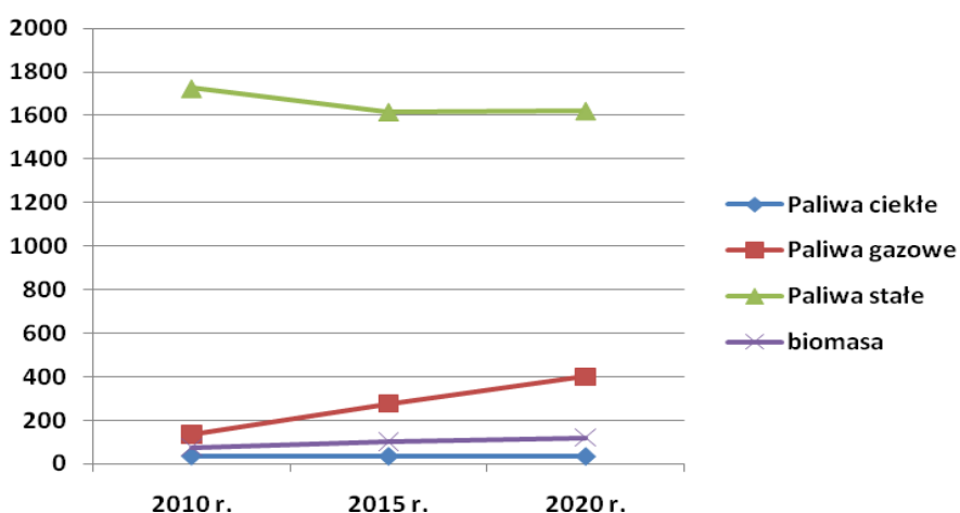
Rysunek 119. Prognoza spalania paliw [PJ] w produkcji energii elektrycznej i ciepła do roku 2020
