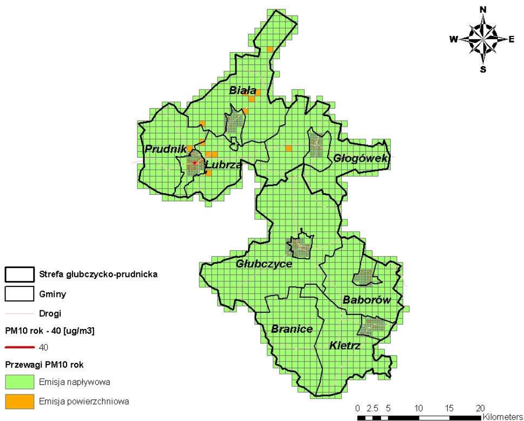
Rysunek 80. Udziały poszczególnych typów emisji w stężeniach pyłu zawieszonego PM 10 o okresie uśredniania wyników pomiarów rok kalendarzowy na terenie strefy głubczycko-prudnickiej w 2008 r.
