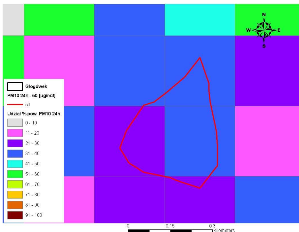
Rysunek 93. Udział procentowy emisji powierzchniowej w imisji całkowitej pyłu zawieszonoego PM 10 o okresie uśredniania wyników pomiarów 24 godziny (36 max) w Głogówku
