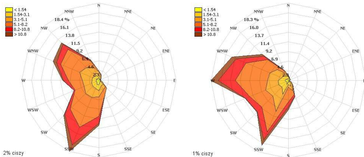
Rysunek 4. Róże wiatrów w oczkach siatki z modelu CALMET zlokalizowanych w Głubczycach i Prudniku w 2008 r.
