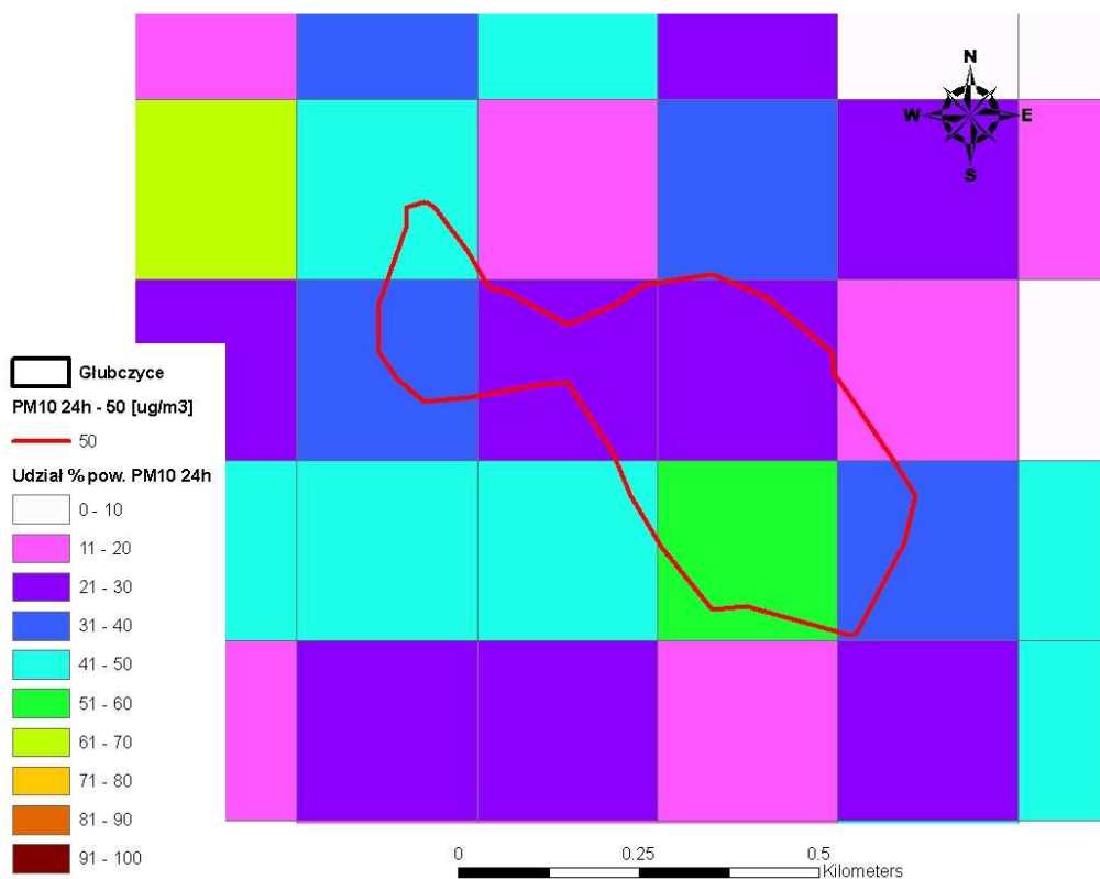
Rysunek 89. Udział procentowy emisji powierzchniowej w imisji całkowitej pyłu zawieszonego PM 10 o okresie uśredniania wyników pomiarów 24 godziny (36 max) w Głubczycach
