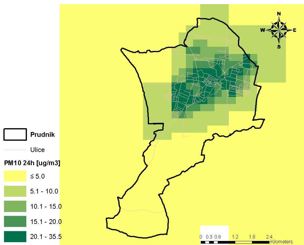
Rysunek 115. Rozkład stężeń pyłu zawieszonego PM 10 o okresie uśredniania wyników pomiarów 24 godziny pochodzących od emisji powierzchniowej , po zastosowaniu działań dot. zmiany ogrzewania w Prudniku
