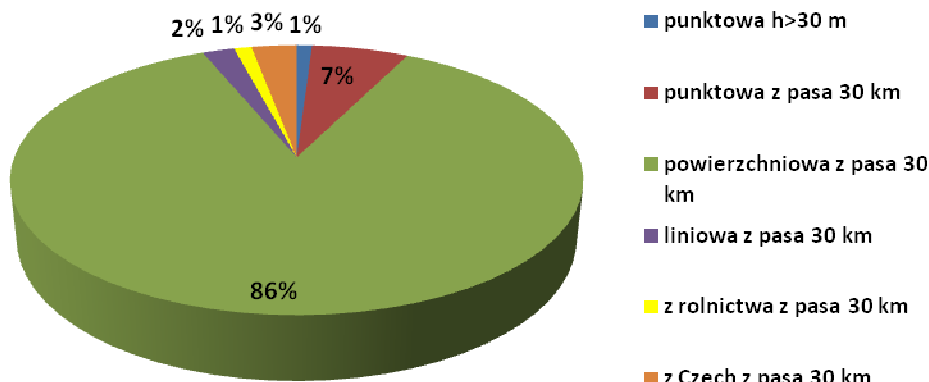
Rysunek 14. Udział procentowy poszczególnych typów emisji pyłu zawieszonego PM 10 w emisji napływowej w strefie głubczycko-prudnickiej w 2008 r.
