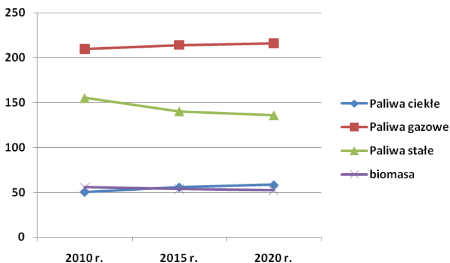
Rysunek 120. Prognoza spalania paliw [PJ] w produkcji przemysłowej i budownictwie do roku 2020
