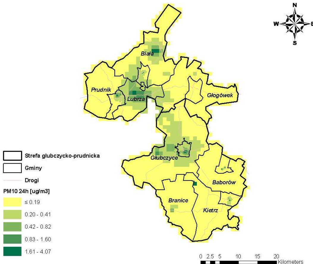
Rysunek 49. Rozkład stężeń pyłu zawieszonego PM 10 o okresie uśredniania wyników pomiarów 24 godziny (36 max) pochodzących od emisji punktowej na terenie strefy głubczycko-prudnickiej w 2008 r.
