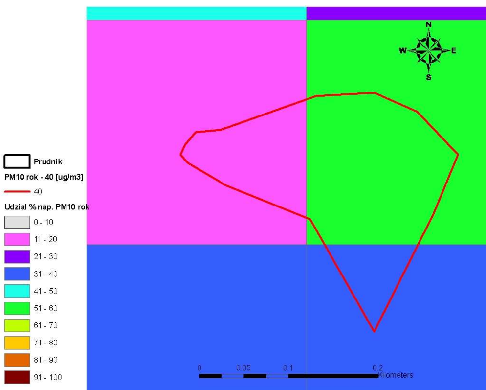
Rysunek 108. Udział procentowy emisji napływowej w imisji całkowitej pyłu zawieszonego PM 10 o okresie uśredniania wyników pomiarów rok kalendarzowy w Prudniku
