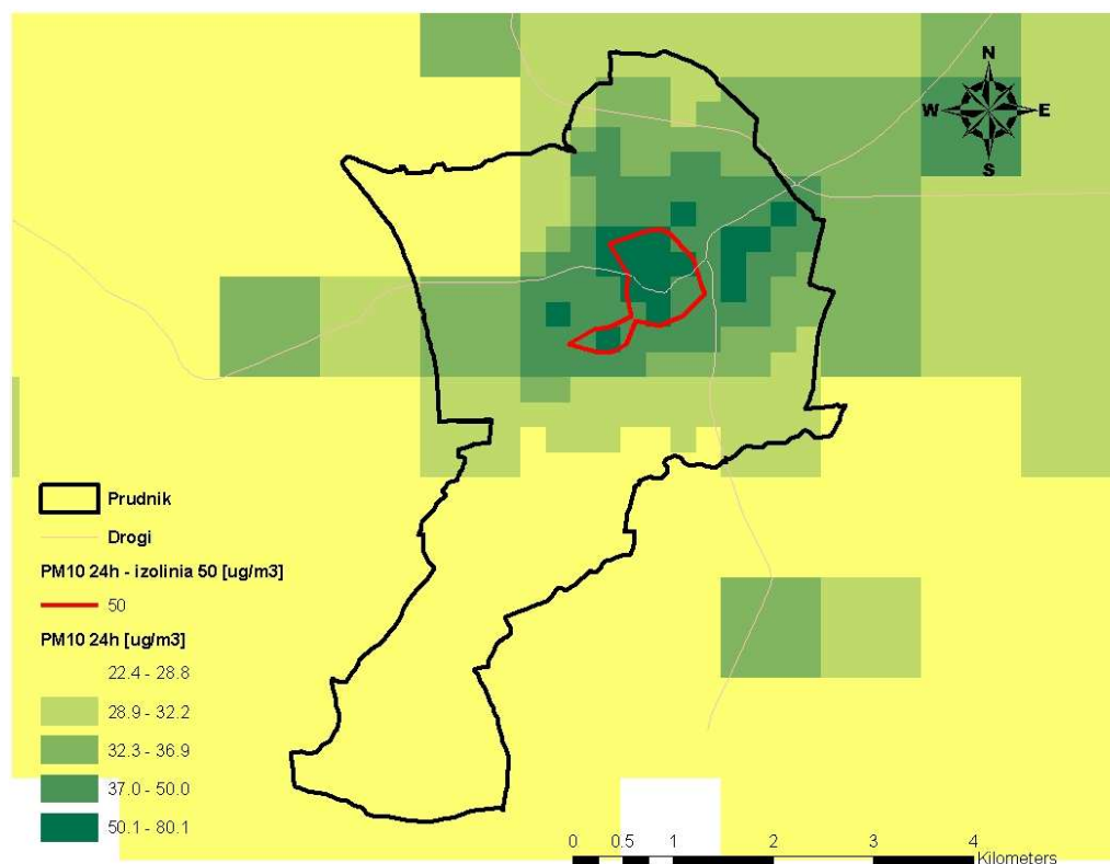
Rysunek 110 Rozkład stężeń pyłu zawieszonego PM 10 o okresie uśredniania wyników pomiarów 24 godziny (36 max) z emisji całkowitej na terenie Prudnika w 2008 r. po odjęciu napływu stężeń pochodzących od emisji naturalnej
