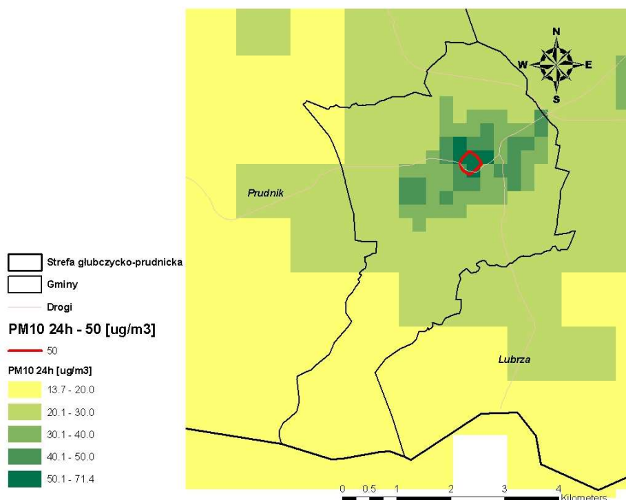
Rysunek 113. Rozkład stężeń pyłu zawieszonego PM 10 o okresie uśredniania wyników pomiarów 24 godziny (36 max) z emisji całkowitej na terenie Prudnika w 2008 r. po odjęciu napływu transgranicznego i stężeń pochodzących od emisji naturalnej
