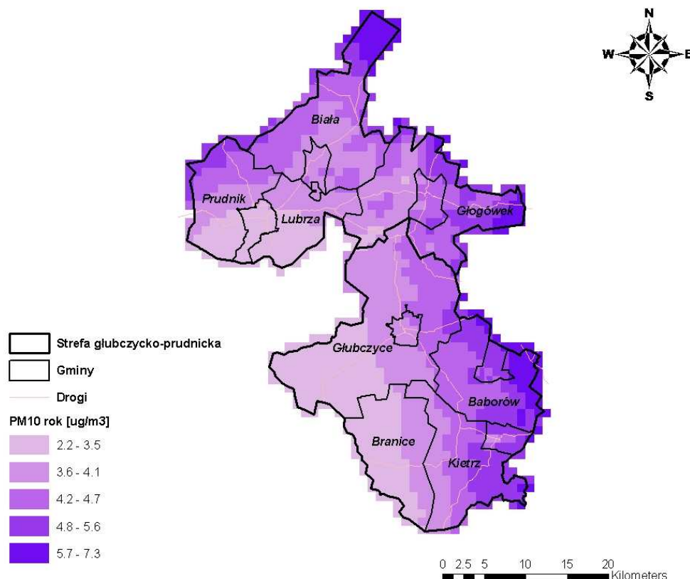
Rysunek 46. Stężenia pyłu zawieszonego PM 10 o okresie uśredniania wyników pomiarów rok kalendarzowy w strefie głubczycko-prudnickiej pochodzące od regionalnej emisji napływowej w 2008 r.
