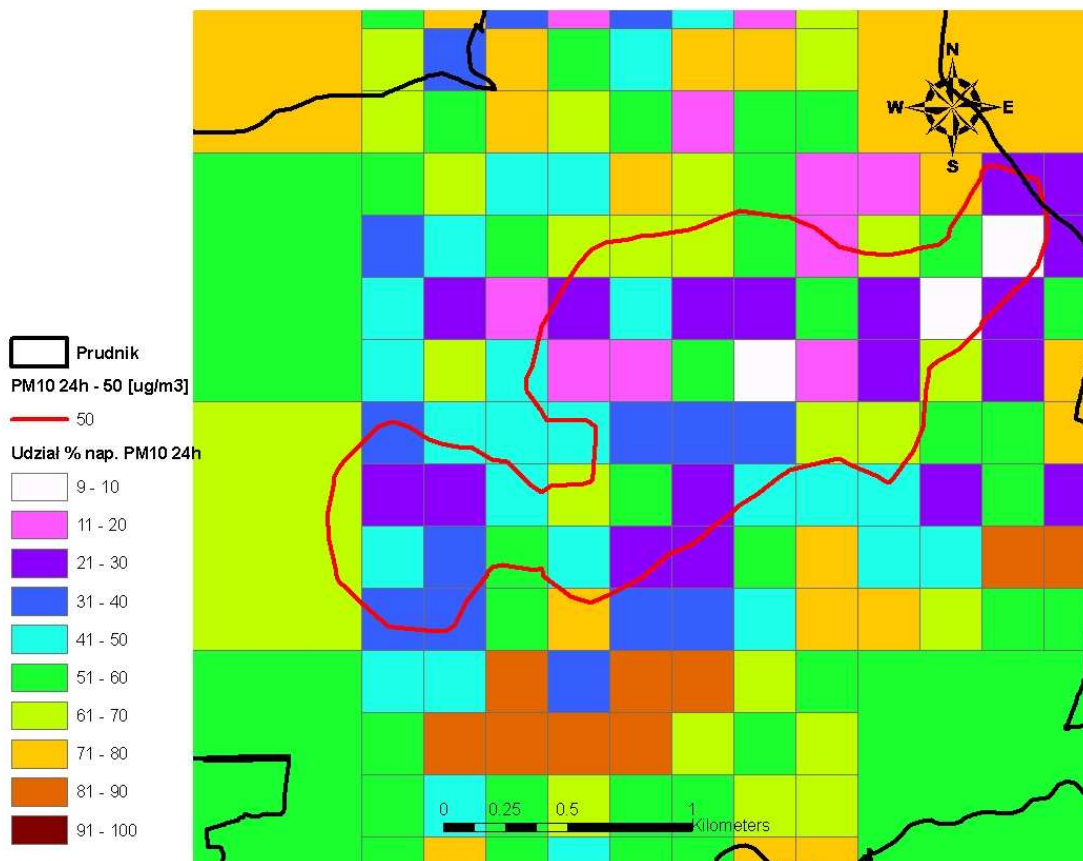
Rysunek 86. Udział procentowy emisji napływowej w imisji całkowitej pyłu zawieszono PM 10 o okresie uśredniania wyników pomiarów 24 godziny (36 max) w Prudniku
