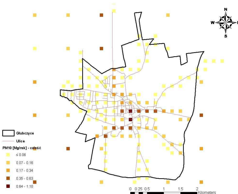
Rysunek 35. Całkowita emisja liniowa pyłu zawieszonego PM 10 w Głubczycach w 2008 r.
