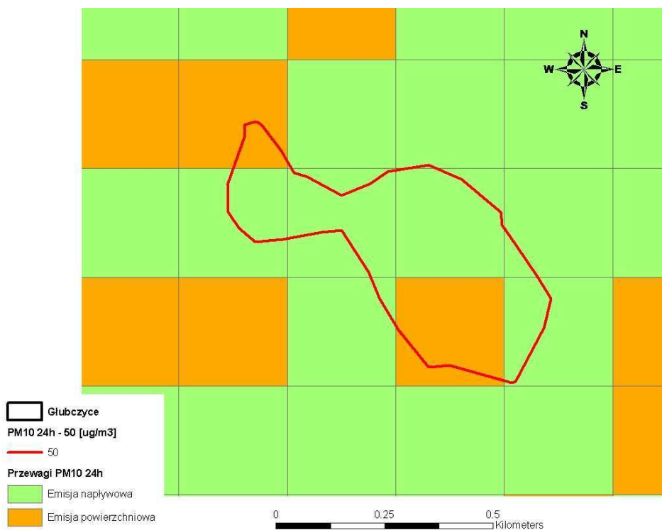
Rysunek 88. Większościowy udział poszczególnych typów emisji w imisji pyłu zawieszono PM 10 o okresie uśredniania wyników pomiarów 24 godziny (36 max) w Głubczycach
