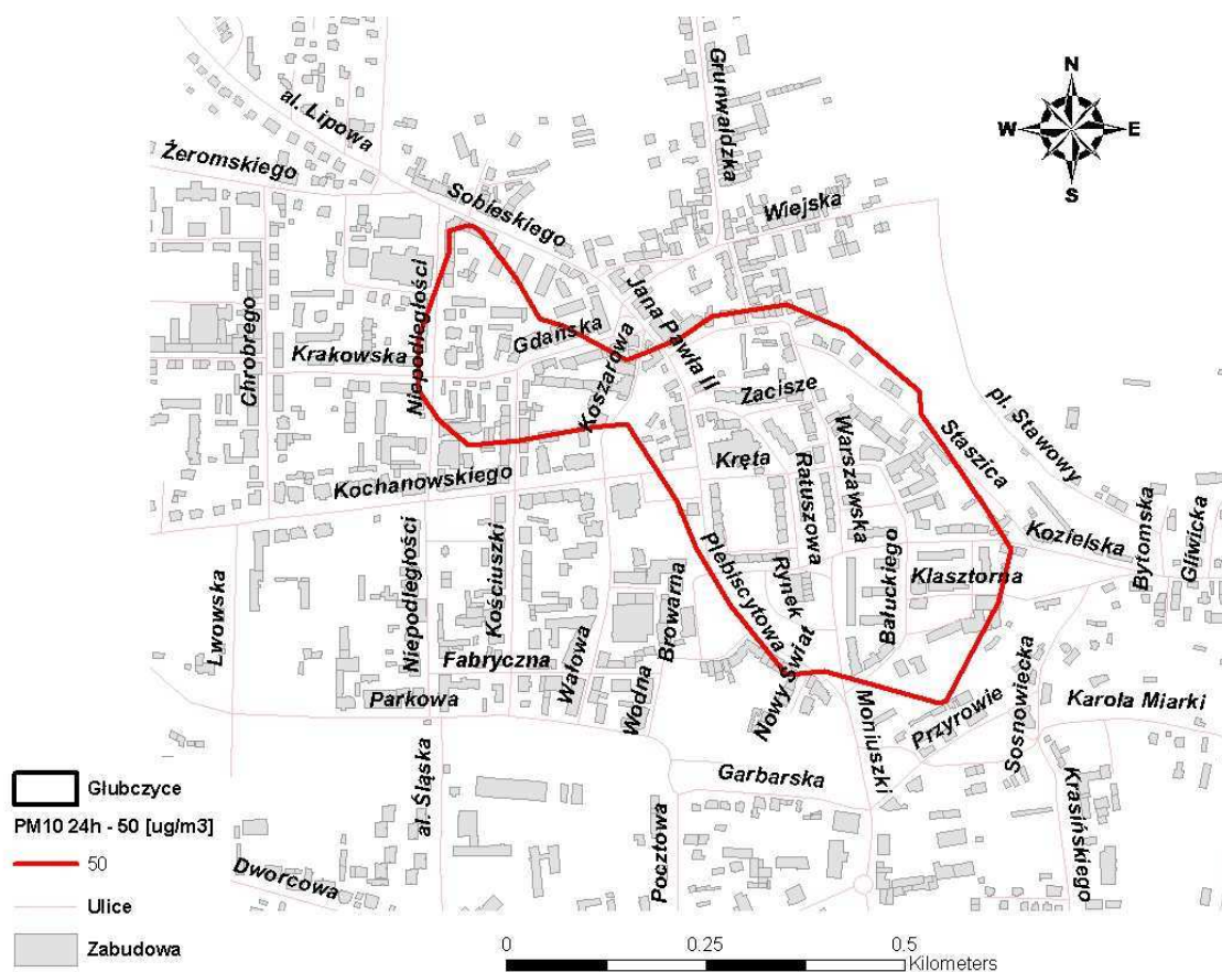
Rysunek 87. Obszar przekroczeń poziomu dopuszczalnego stężeń pyłu zawieszono PM 10 o okresie uśredniania wyników pomiarów 24 godziny (36 max) w Głubczycach
