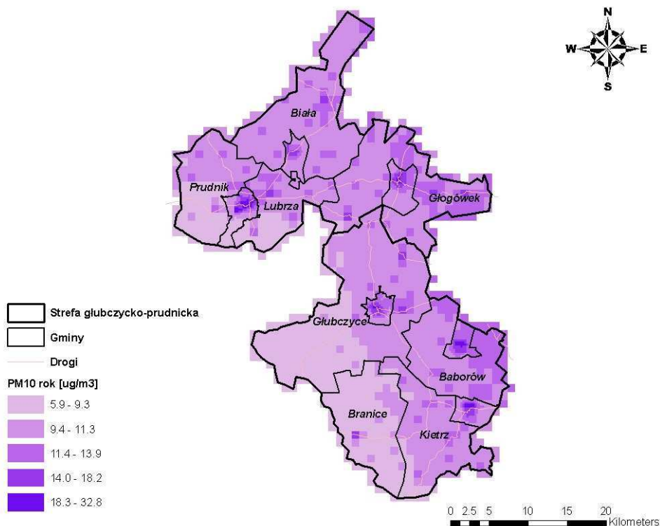
Rysunek 113. Rozkład stężeń pyłu zawieszonego PM 10 o okresie uśredniania wyników pomiarów rok kalendarzowy z emisji całkowitej na terenie strefy głubczycko-prudnickiej w 2008 r. po odjęciu napływu transgranicznego i stężeń pochodzących od emisji naturalnej
