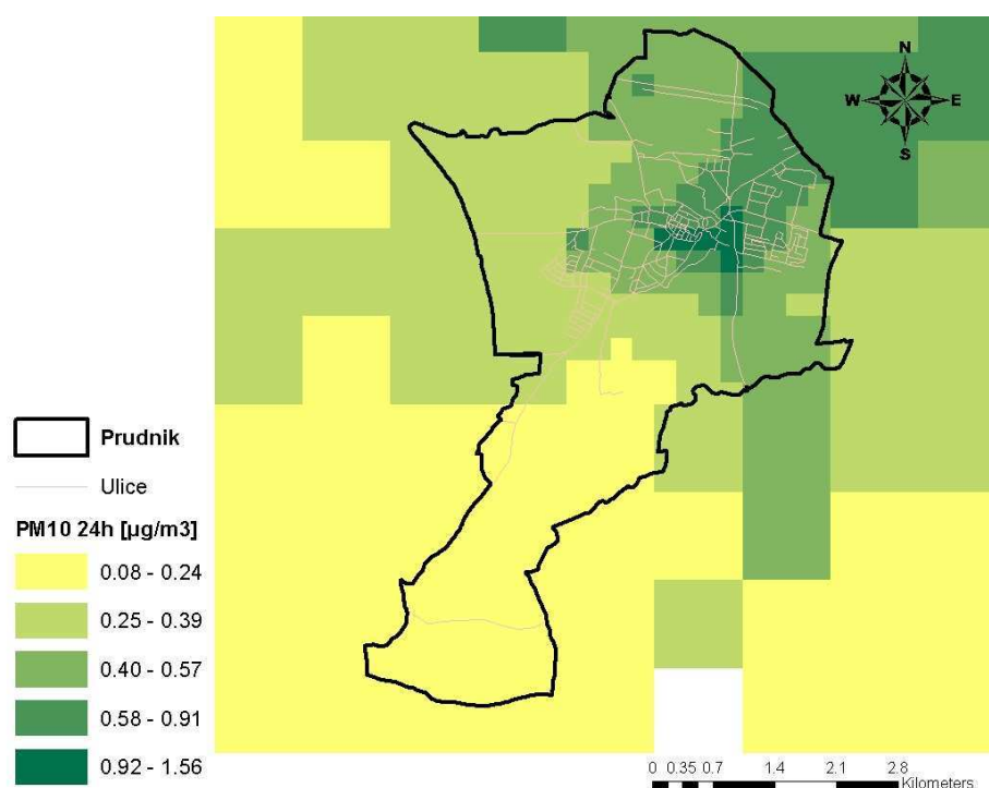
Rysunek 115. Rozkład stężeń pyłu zawieszono PM 10 o okresie uśredniania wyników pomiarów 24 godziny pochodzących od emisji liniowej , po zastosowaniu działań w zakresie komunikacji w Prudniku
