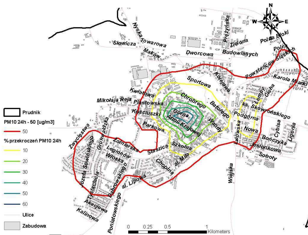
Rysunek 83. Wartość procentowa przekroczeń stężeń pyłu zawieszanego PM 10 o okresie uśredniania wyników pomiarów 24 godziny (36 max) w Prudniku
