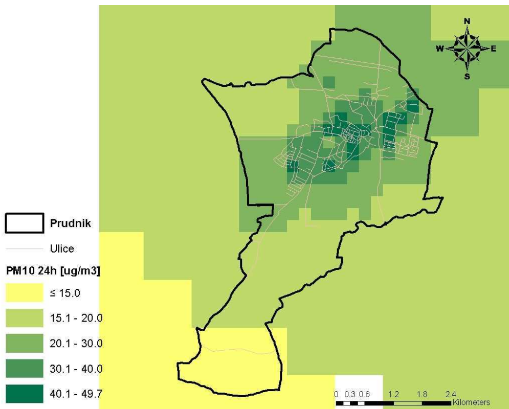
Rysunek 116. Rozkład stężeń pyłu zawieszonego PM 10 o okresie uśredniania wyników pomiarów 24 godziny pochodzących od całkowitej emisji, po zastosowaniu działań naprawczych oraz odjęciu napływu transgranicznego i stężeń pochodzących od emisji naturalnej
